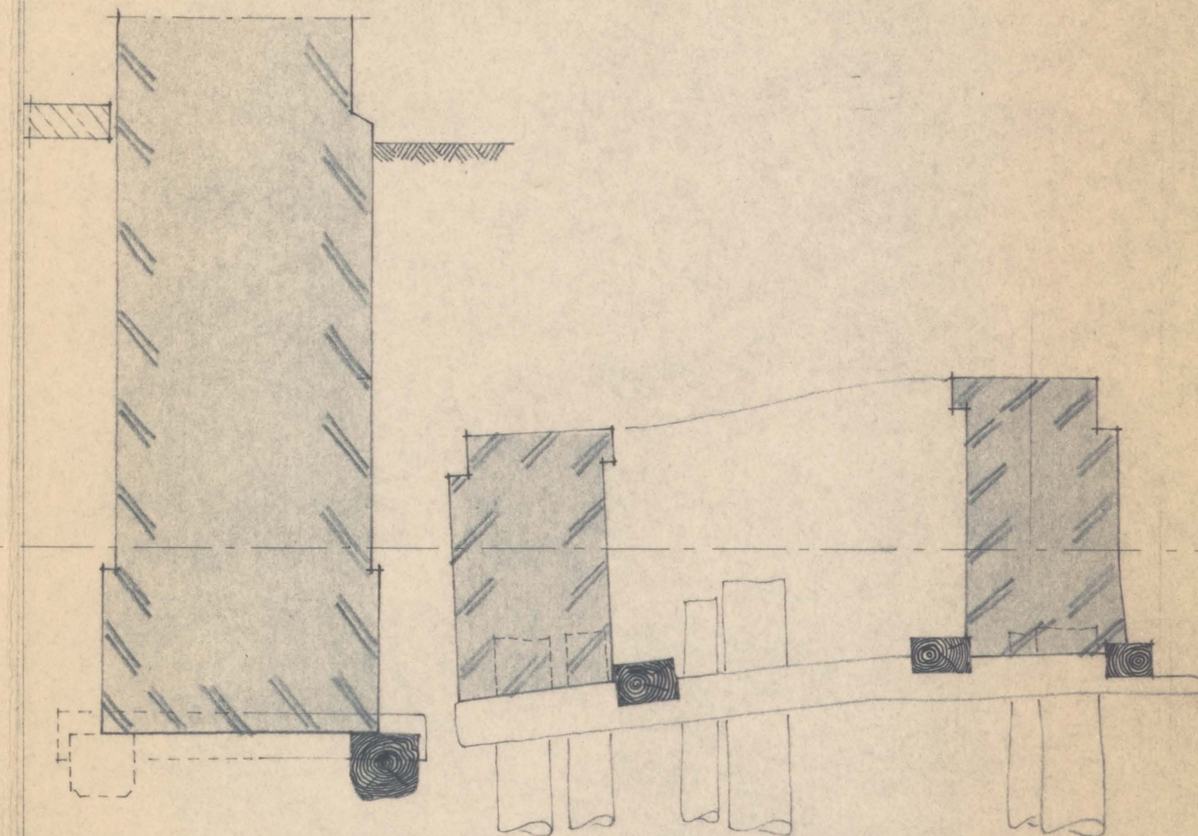
DOORSNEDEN C - C
