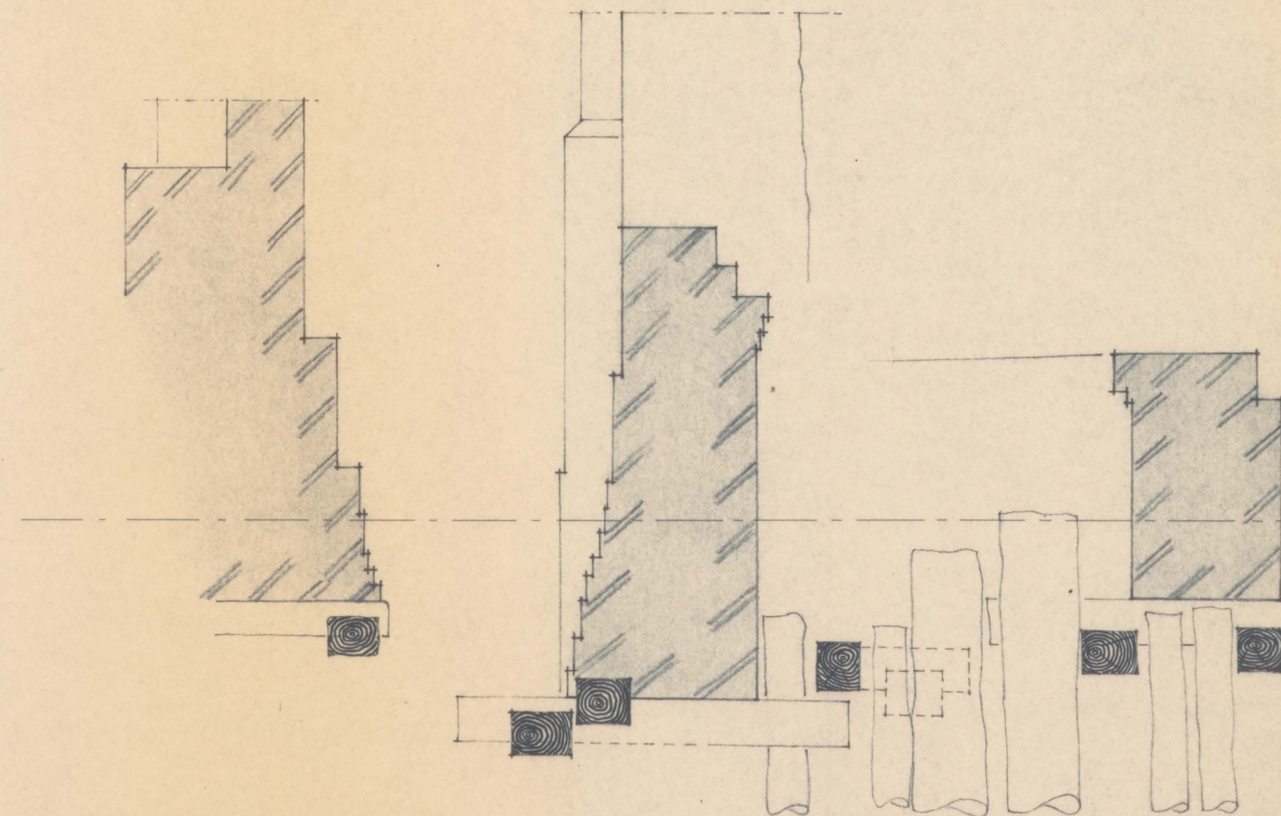
DOORSNEDEN F - F
